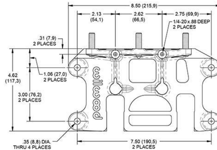
VIEW A-A
